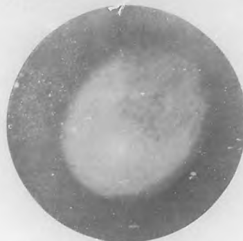
Como una nebulosidad globular con una fuerte condensación central.
