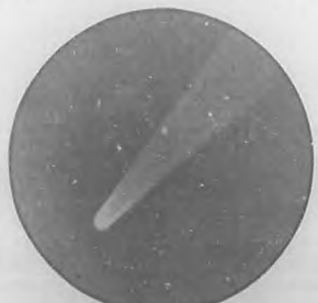
Núcleo brillantísimo muy definido y cola bifurcada y rectilínea.
