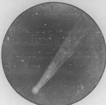
Cabellera contraída y cauda constituida por estrías y aborregados.
